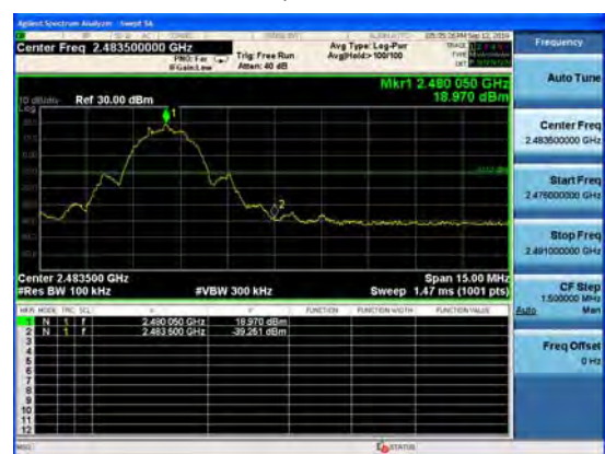
BLE V5.0-125K, Channel No.: 39
