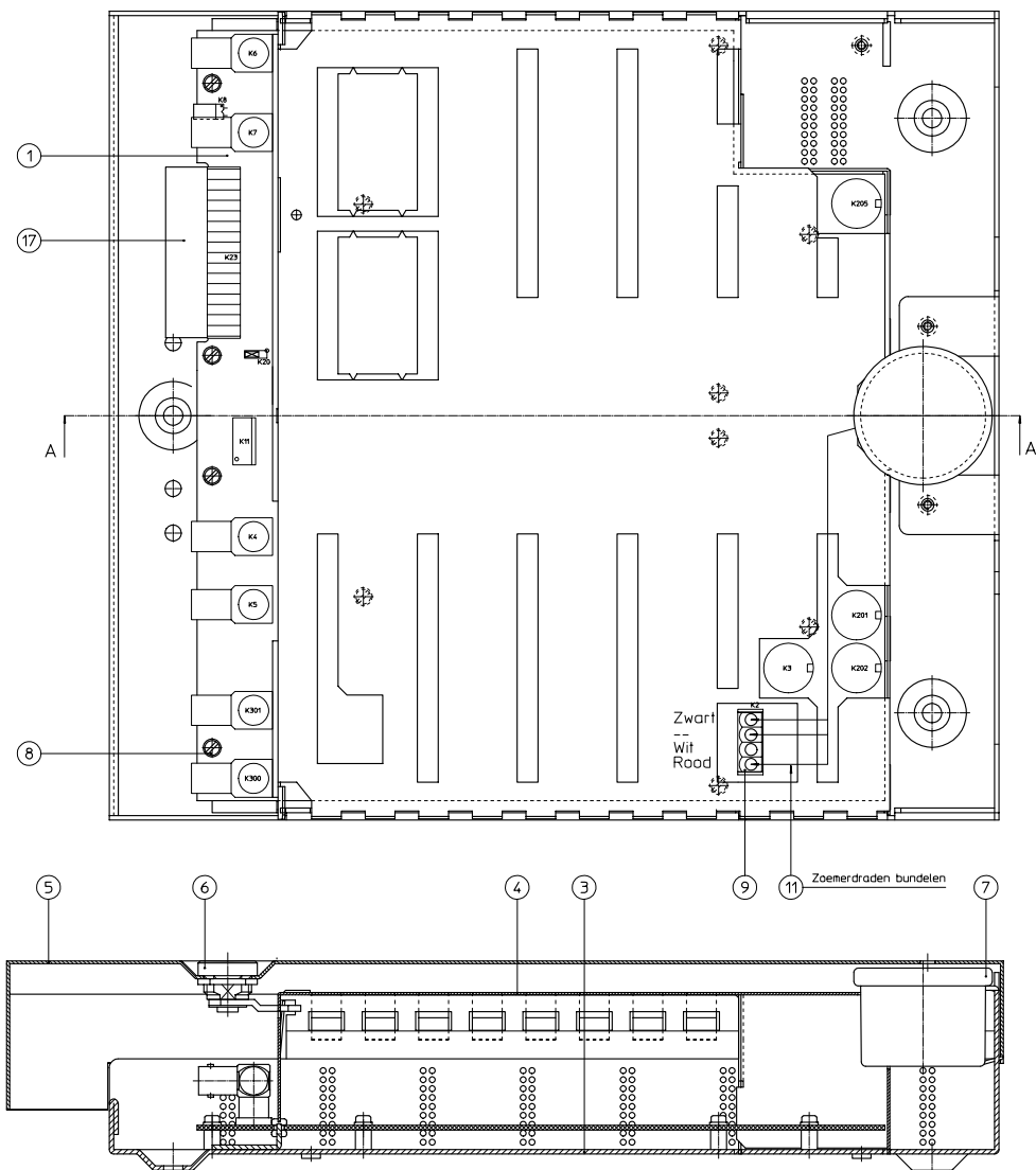
AANZICHT ZONDER DEKSEL ⑤ EN SLOT ⑥
