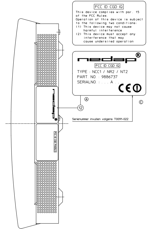
TYPEPLAAT BIJ IQ3E (9886737)
