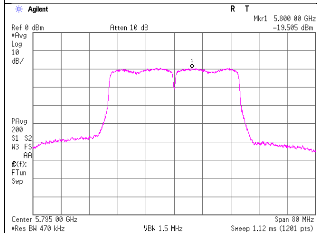
5795MHz
