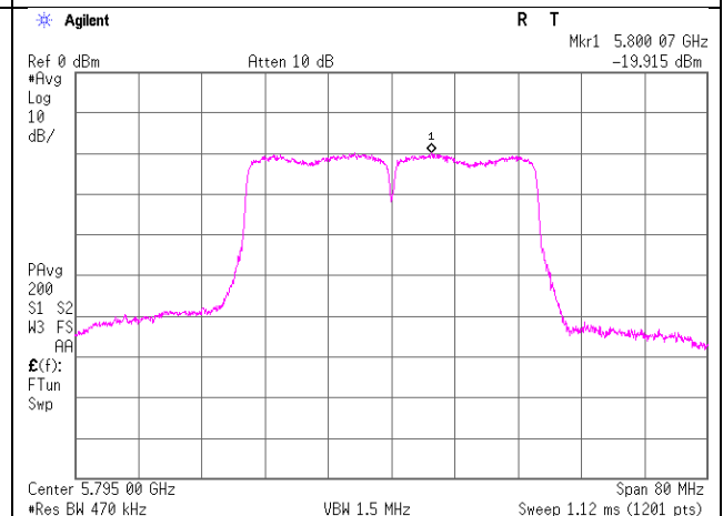
5795MHz
