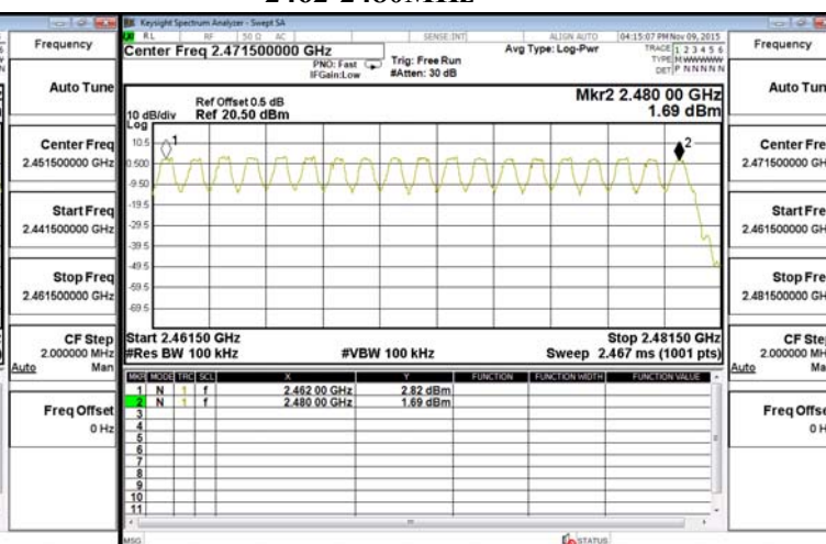
2462-2480MHz
