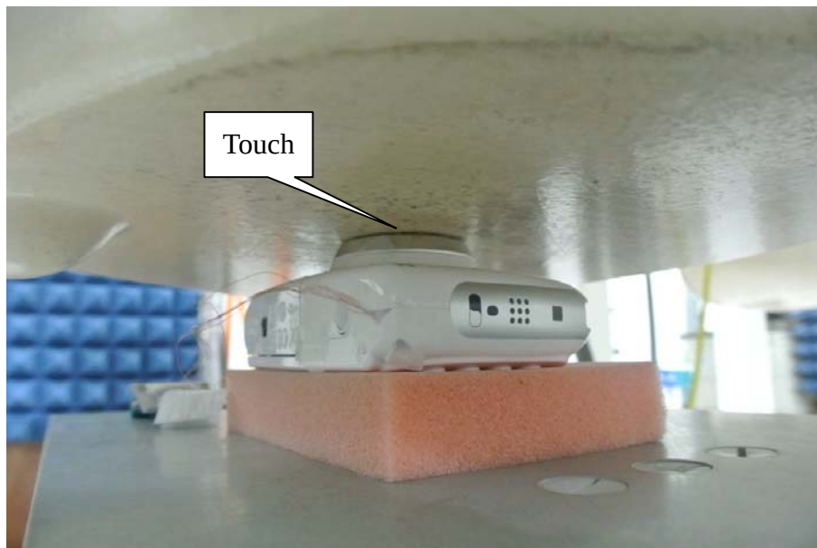
EUT Front
