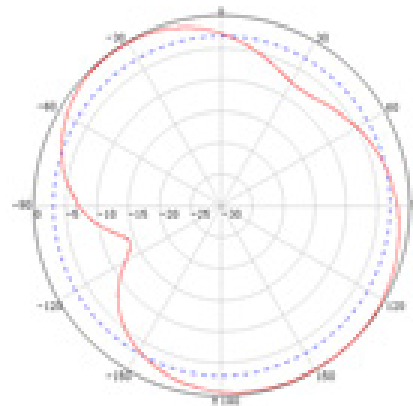
V-Plane
