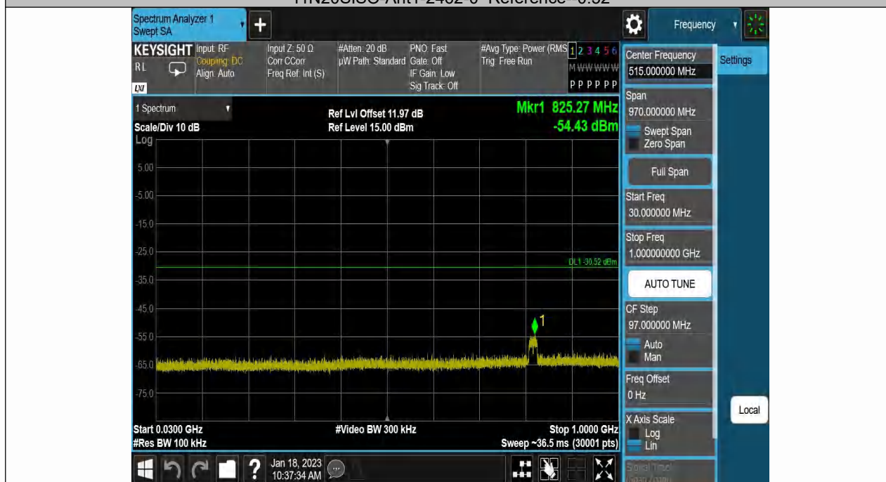
11N20SISO-Ant1-2462-30~1000--0.52
