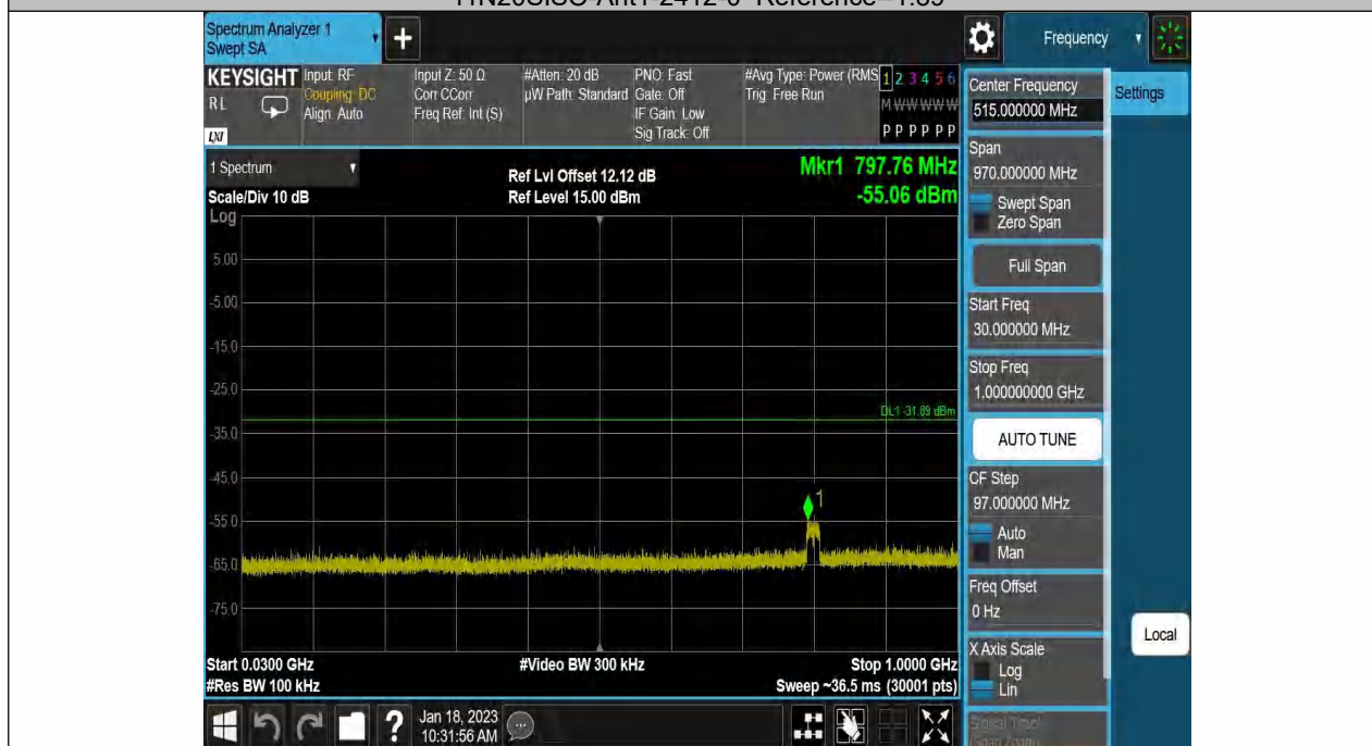
11N20SISO-Ant1-2412-30~1000--1.89
