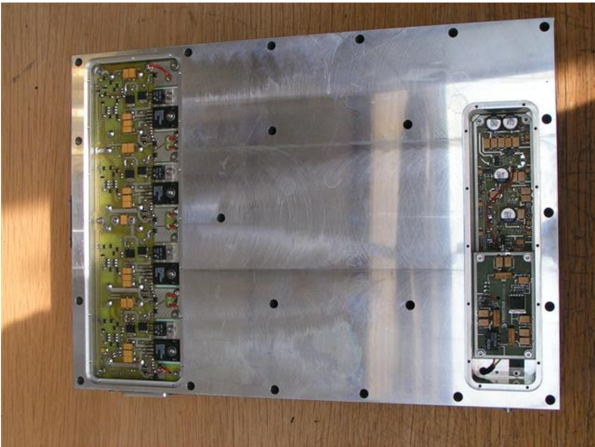
DTX-A213 HPA DC
