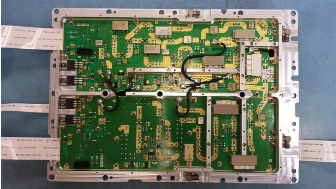
DTX-A213 DOWNCONVERTER
