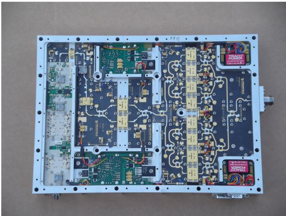
DTX-A213 HPA RF
