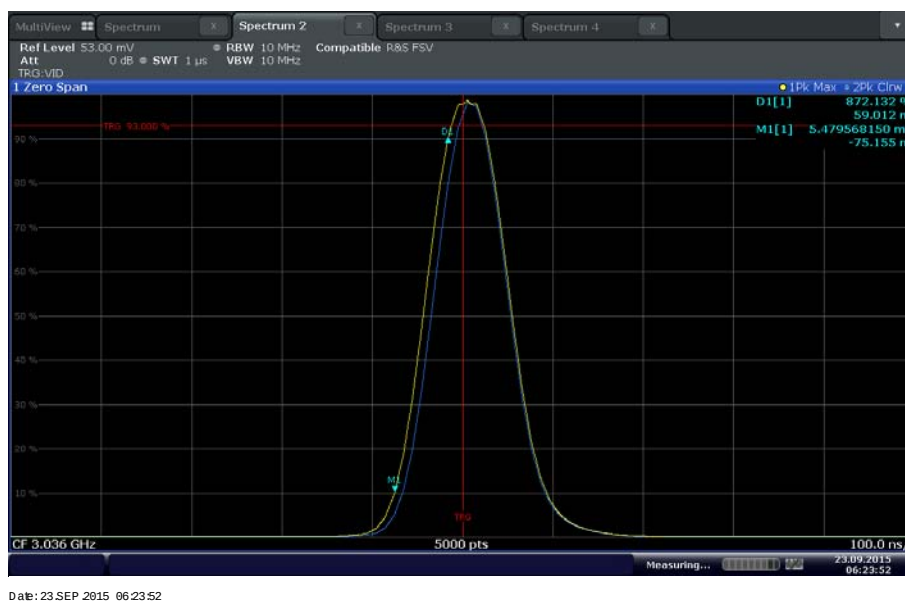
PON SP1 Pulse Rise Time
