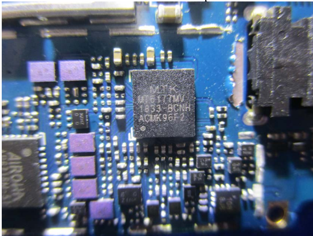
GSM&WCDMA&LTE Chip
