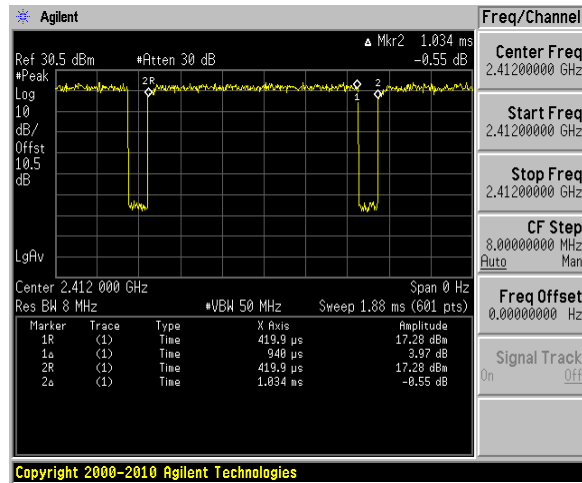
802.11n40 mode
