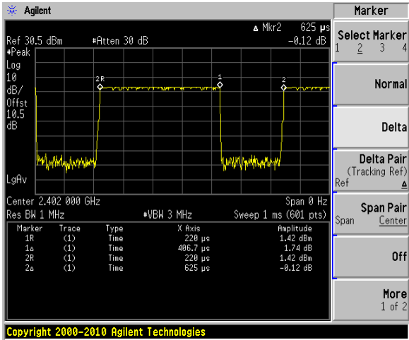
BLE
