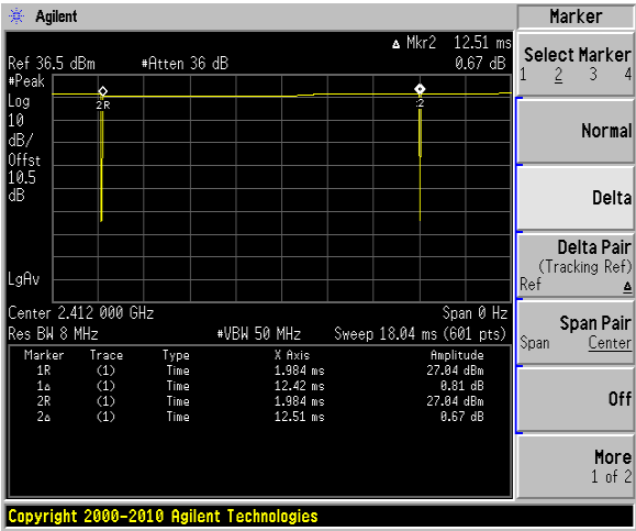
802.11b mode
