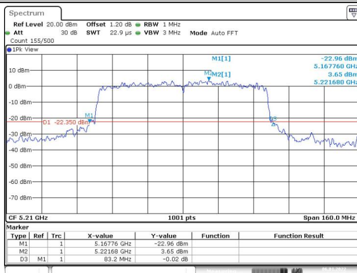
11AC80SISO_Ant1_5210
