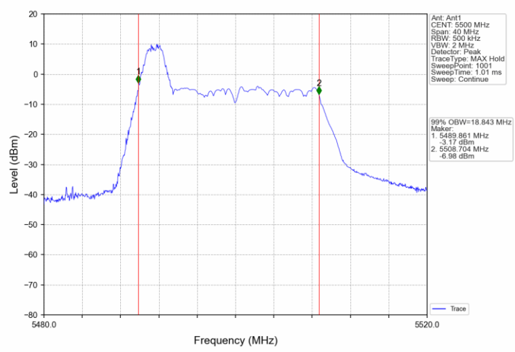
802.11ax(HEW20)_LCH_5500MHz_RU52_37_Ant1_NTNV
