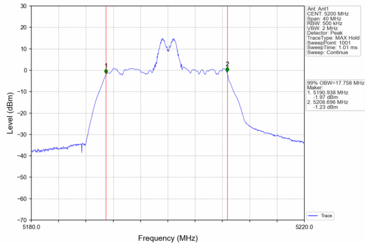
802.11ax(HEW20) MCH 5200MHz RU52_38 Ant1 NTNv
