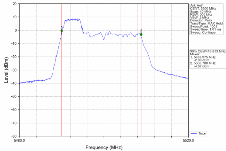
802.11ax(HEW20) LCH 5500MHz RU106 53 Ant1 NTNv
