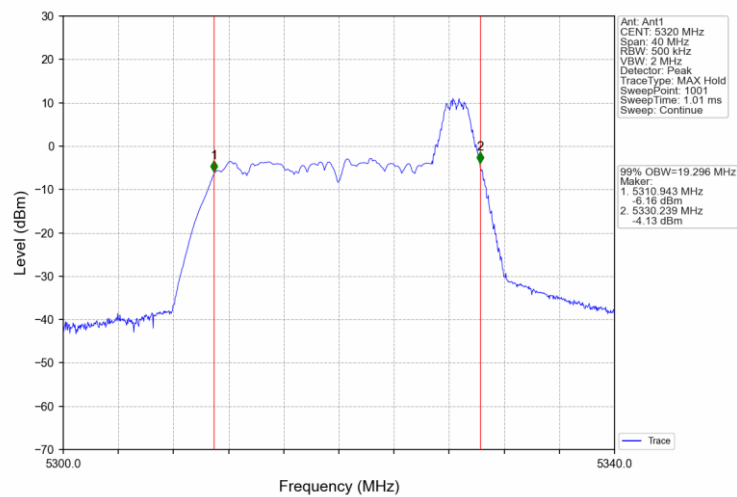
802.11ax(HEW20)_HCH_5320MHz_RU52_40_Ant1_NTNV
