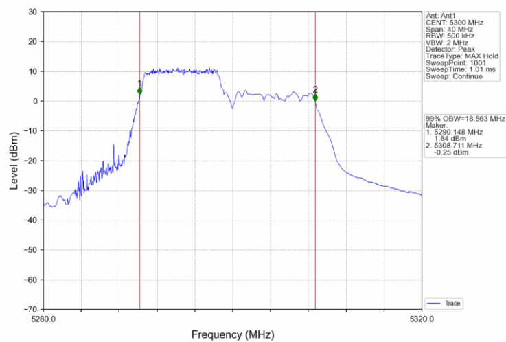
802.11ax(HEW20) MCH 5300MHz RU242_61 Ant1 NTNv
