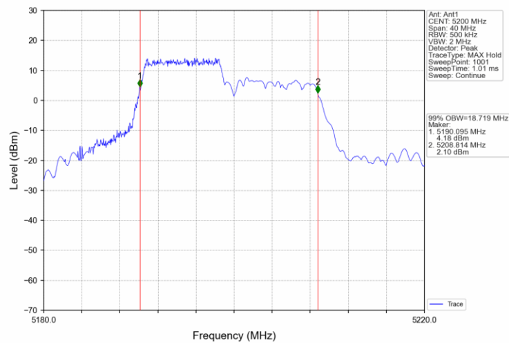
802.11ax(HEW20) MCH 5200MHz RU242_61 Ant1 NTNv
