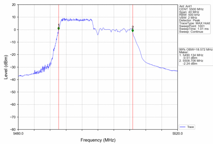
802.11ax(HEW20) LCH 5500MHz RU242 61 Ant1 NTNv
