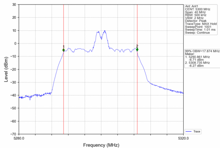
802.11ax(HEW20) MCH 5300MHz RU52_38 Ant1 NTNv
