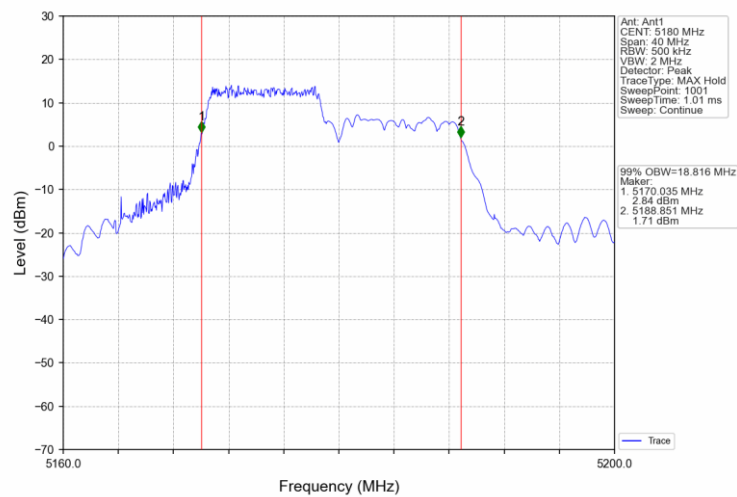
802.11ax(HEW20) LCH 5180MHz RU242_61 Ant1 NTNv
