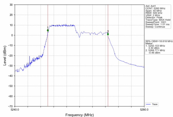
802.11ax(HEW20) LCH 5260MHz RU242_61 Ant1 NTNv
