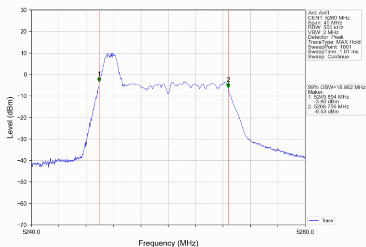
802.11ax(HEW20)_LCH_5260MHz_RU52_37_Ant1_NTNV
