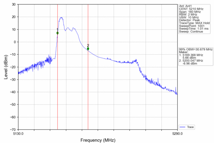
802.11ax(HEW80)_MCH_5210MHz_RU106_53_Ant1_NTNV
