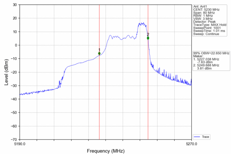
802.11ax(HEW40)_HCH_5230MHz_RU106_56_Ant1_NTNV
