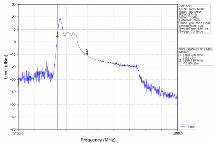
802.11ax(HEW80)_MCH_5210MHz_RU52_37_Ant1_NTNV
