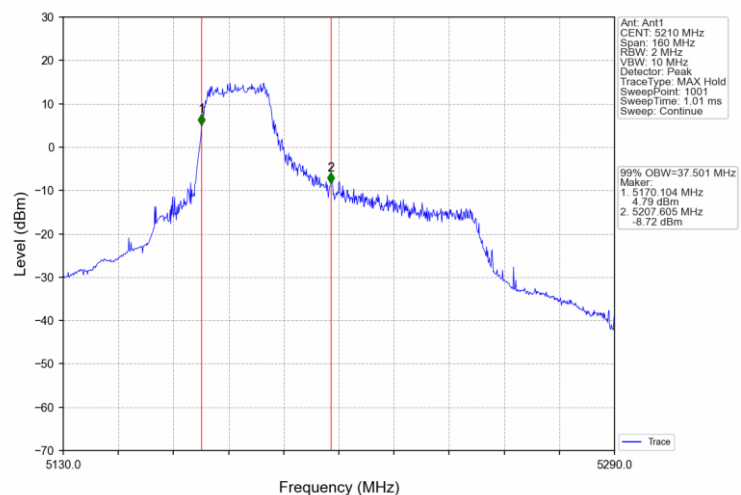
802.11ax(HEW80)_MCH_5210MHz_RU484_65_Ant1_NTNV
