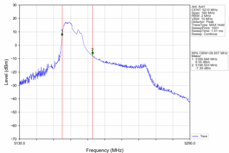
802.11ax(HEW80)_MCH_5210MHz_RU242_61_Ant1_NTNV
