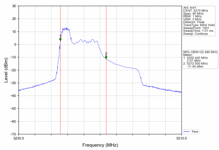
802.11ax(HEW40) LCH 5270MHz RU106_53 Ant1 NTNv
