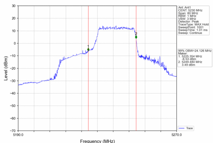
802.11ax(HEW40)_HCH_5230MHz_RU484_65_Ant1_NTNV
