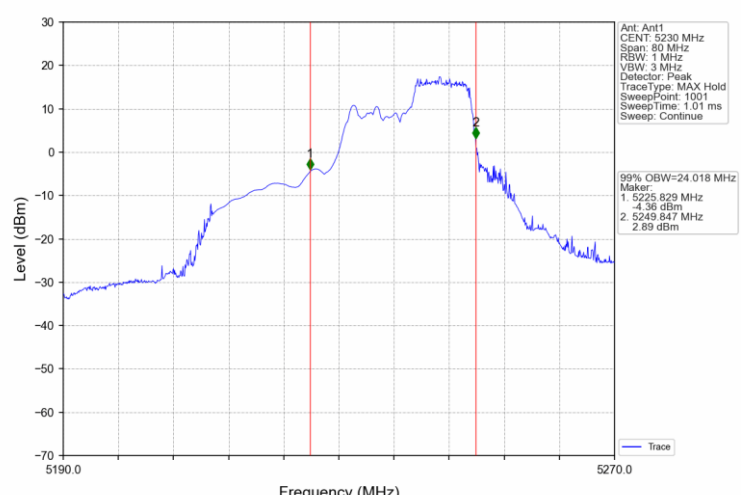
802.11ax(HEW40)_HCH_5230MHz_RU242_62_Ant1_NTNV
