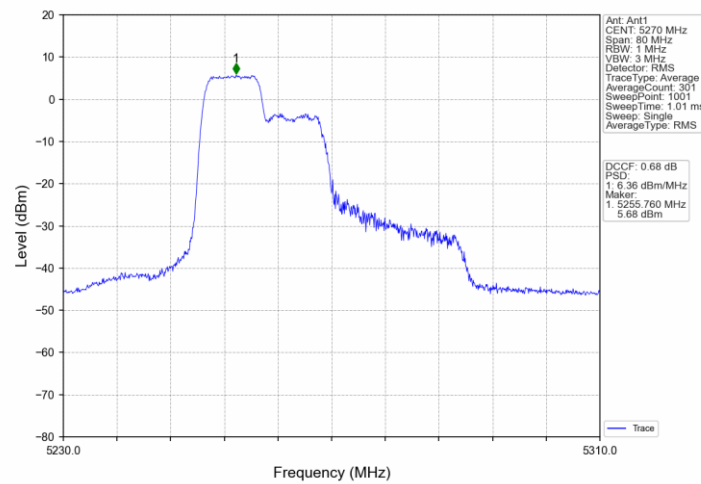
802.11ax(HEW40)_LCH_5270MHz_RU242_61_Ant1_NTNV
