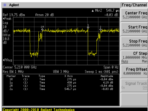
802.11ac80 mode
