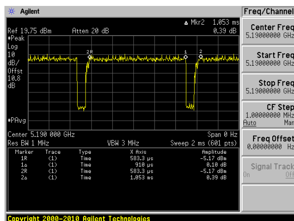
802.11n40 mode
