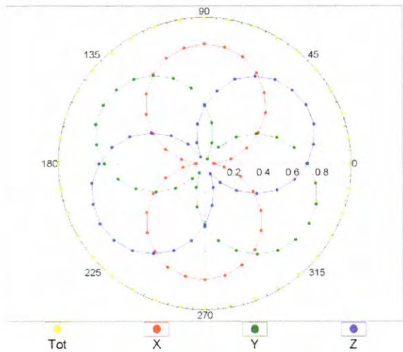
f=450 MHz,TEM
