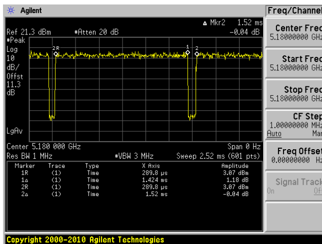
802.11a mode
