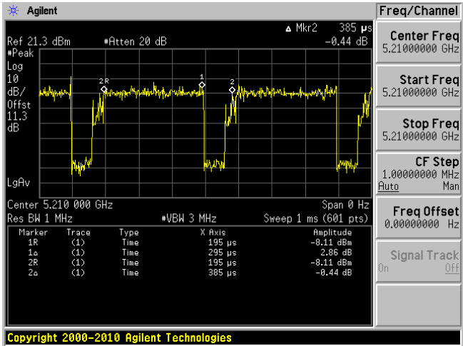
802.11ac80 mode
