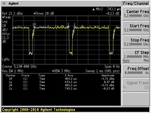
802.11ac40 mode
