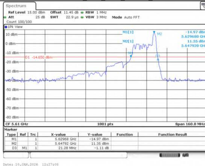
11AX80SISO Ant1 5610 52Tone RU52
