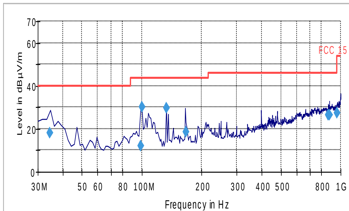
FCC 15 30-1000MHz
