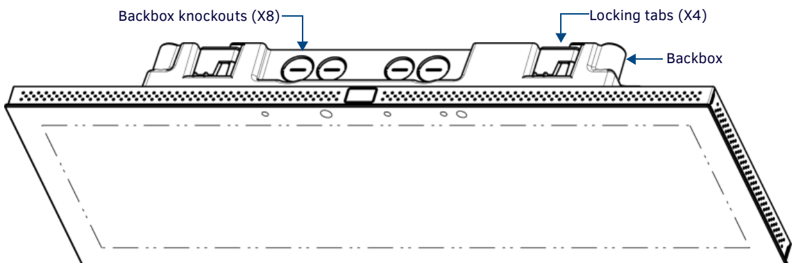
FIG. 24 MXD-1900L-PAN (Landscape)
