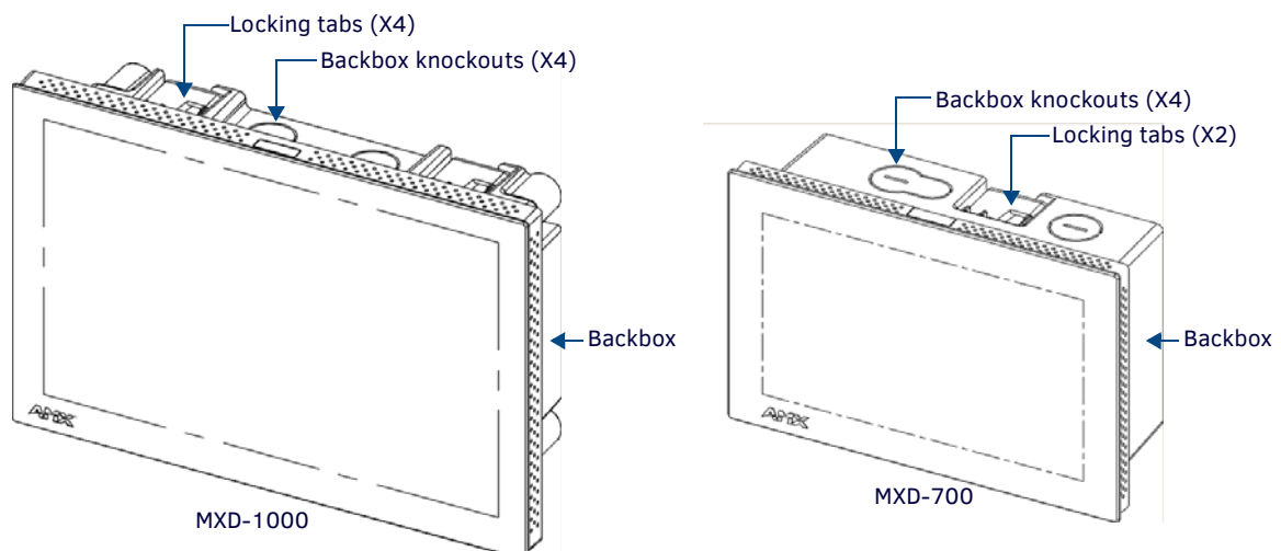
FIG. 37 MXD-1000 and MXD-700 (Landscape)
