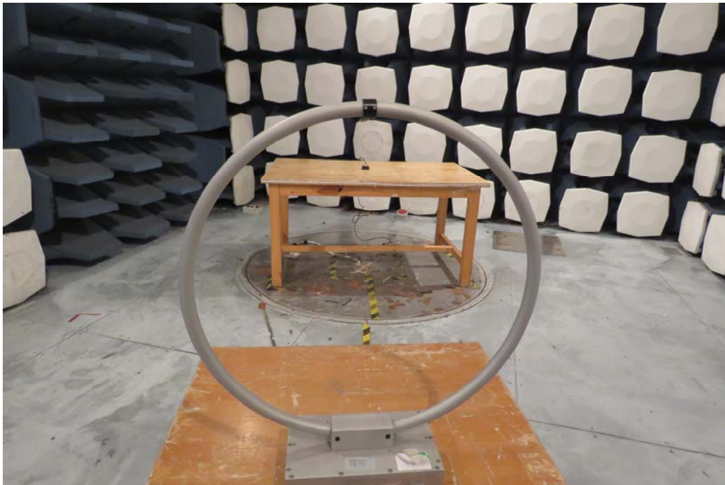
9kHz-30MHz
