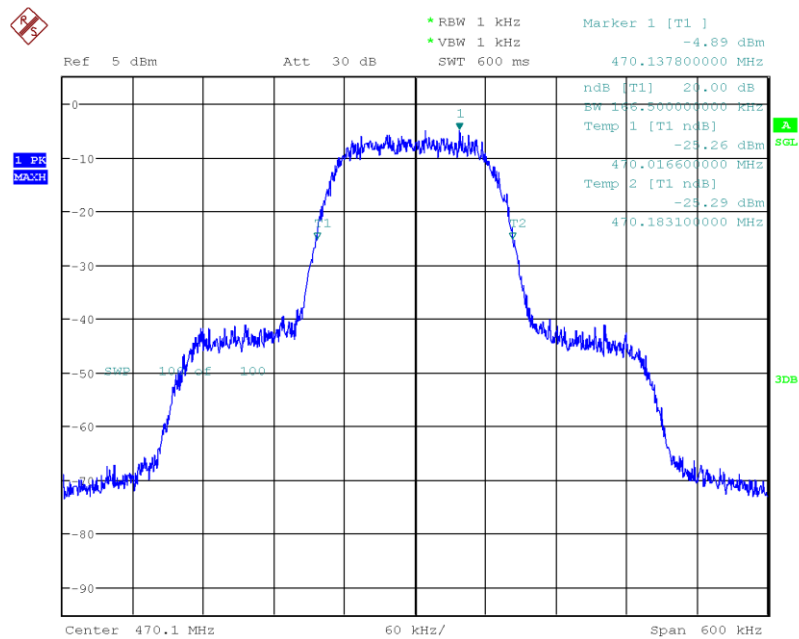
Normal Voltage, -30°C, D2 mode, 470.100 MHz
