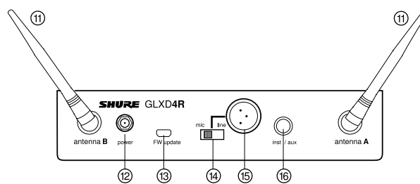
Panneau arrière
