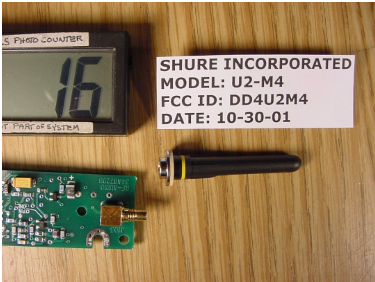
Antenna
