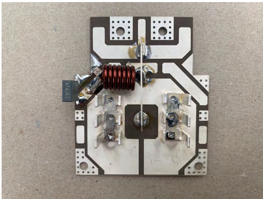
MAMP9A224-0 SCHEDA MODULO OUT 61K25 2KW TOP
