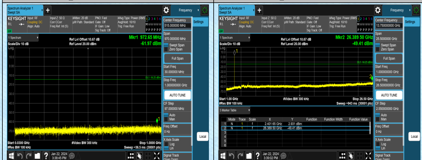
BLE_2M-Ant1-2402-30~1000
