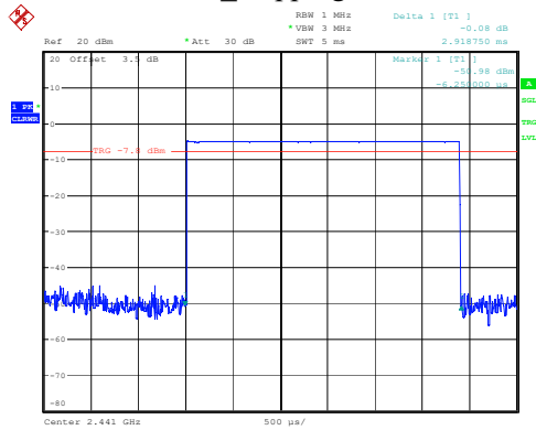
DH5_Hopping 2.919ms
