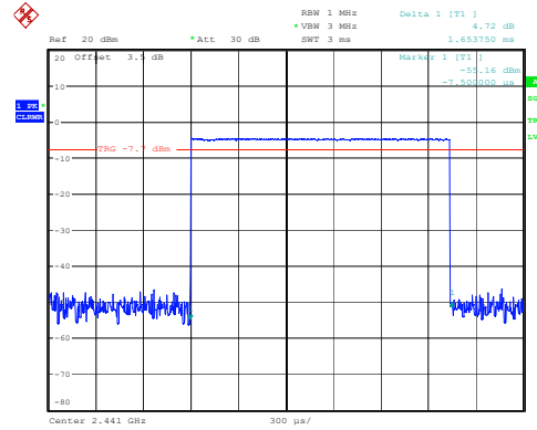
DH3_Hopping 1.654ms
