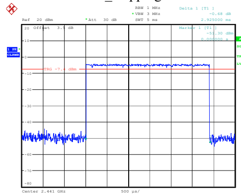
2DH5_Hopping 2.925ms
