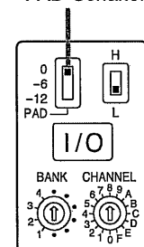
PAD-Schalter
