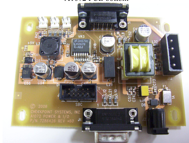
A1072 PCB top
