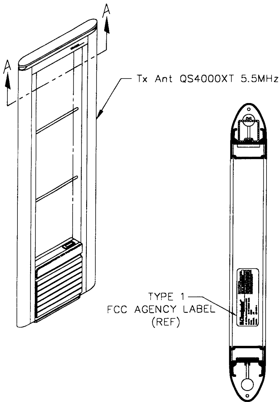
SECTION A-A SCALE: 2/1
