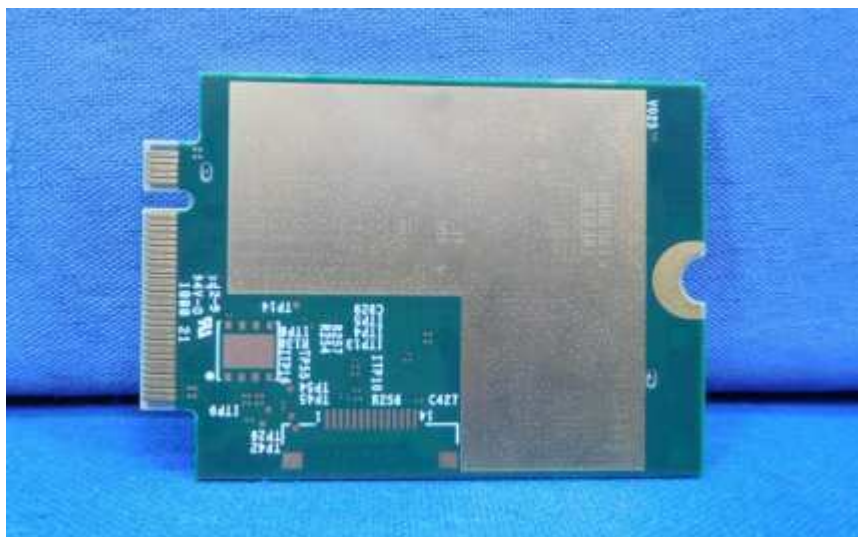
Module Back
