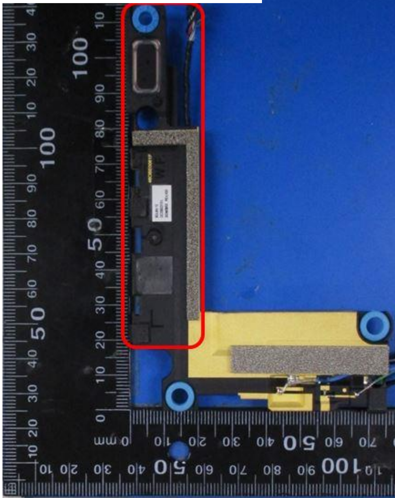
WWAN Aux &amp; GNSS L1 Antenna for Wistron NeWeb Corp.
