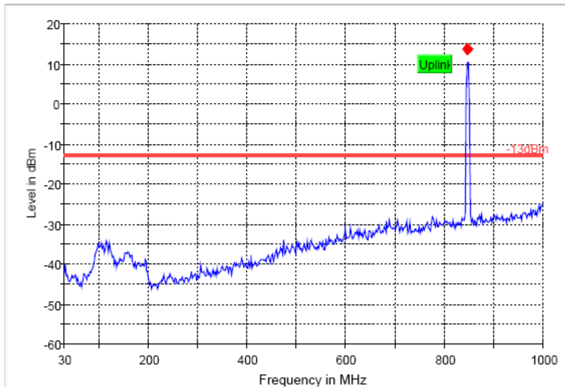
FCC 22 30-1000MHz
