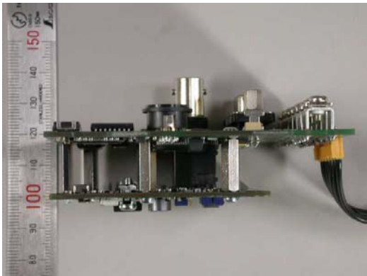
PWB(1)-PWB(2) Side
