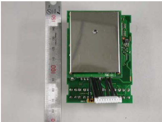
PWB(1)-PWB(2) Front
