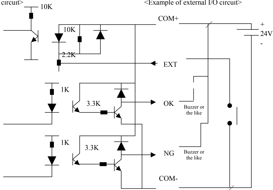
&lt;External I/O circuit&gt;
