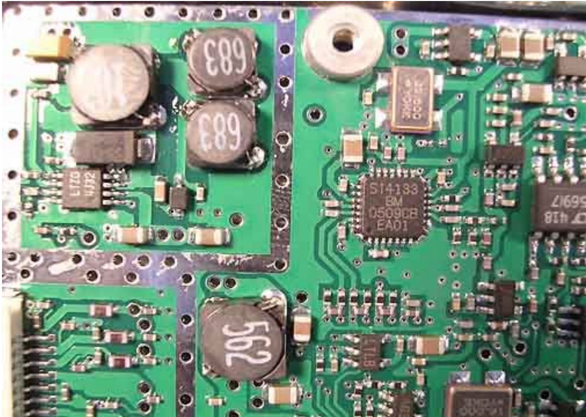
RFID Reader Module Inside 1
