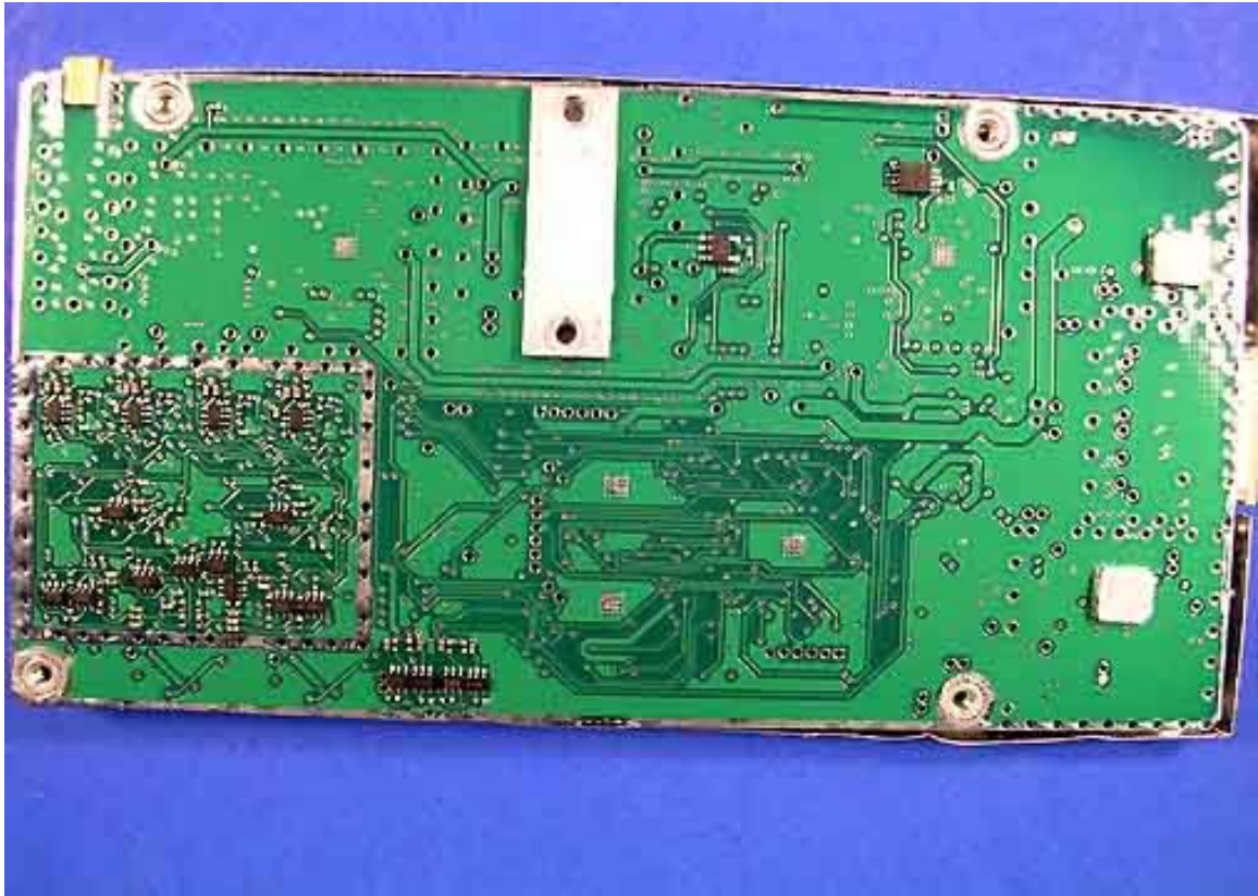
RFID Reader Module Back
