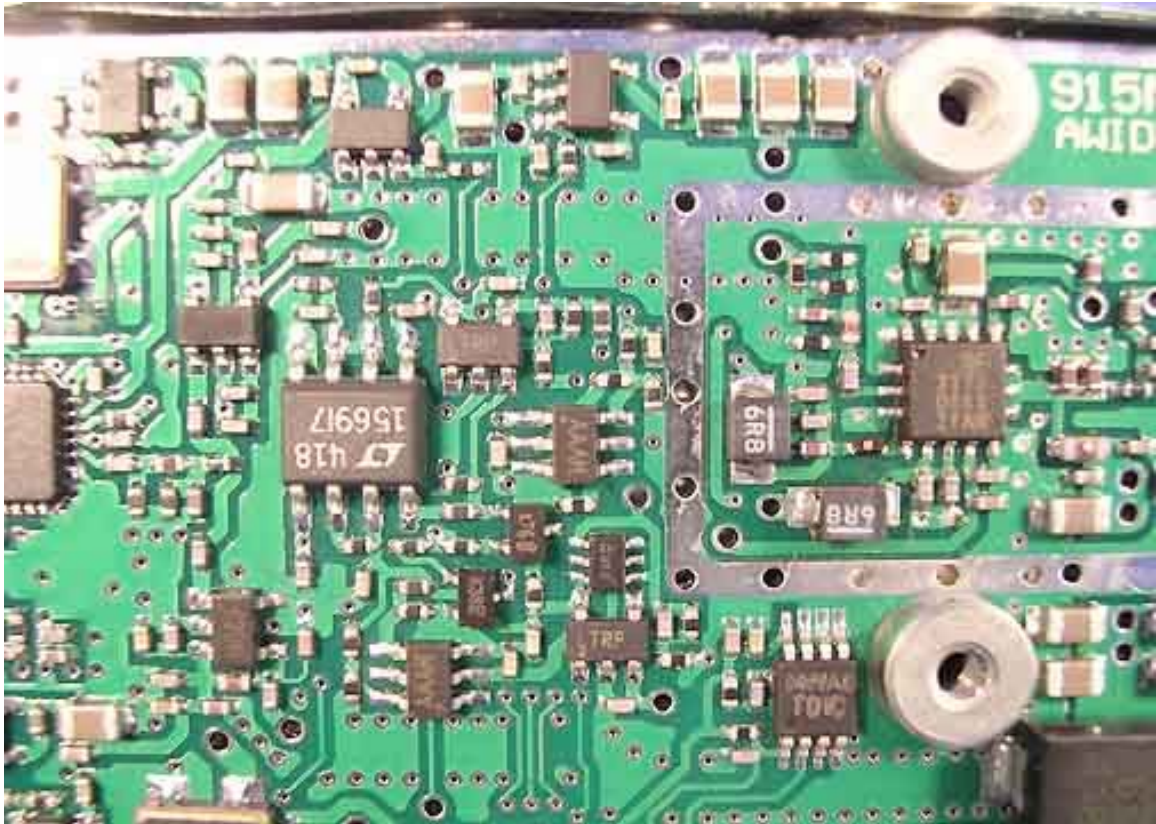
RFID Reader Module Inside 3
