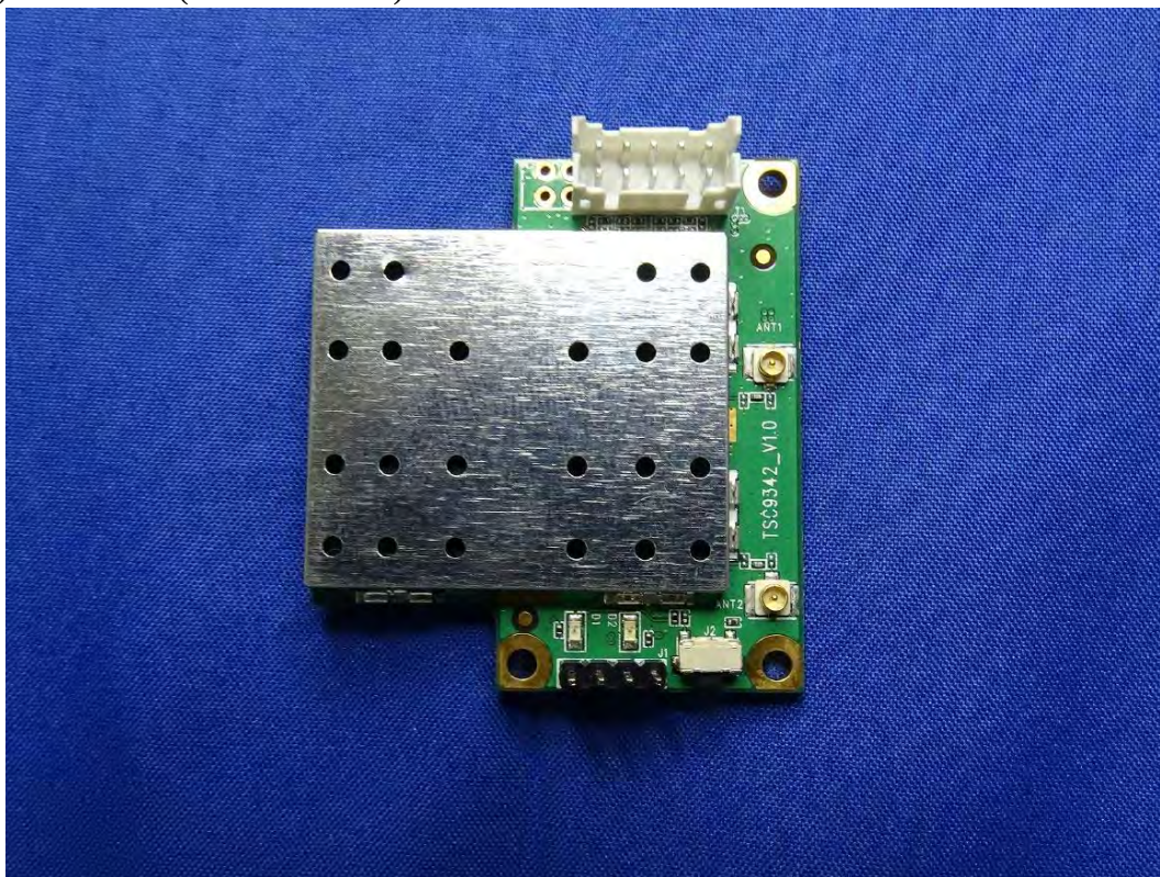
(13) EUT Photo (WLAN Module)
