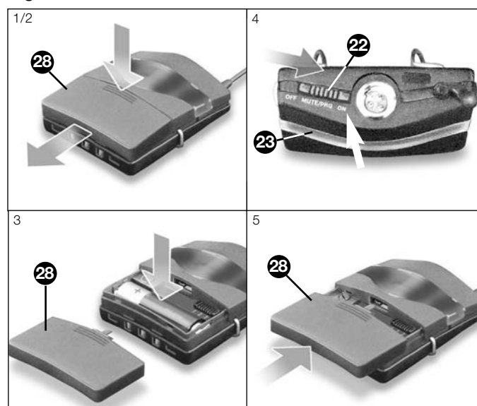
Fig. 8 / PT 40 FLEXX
