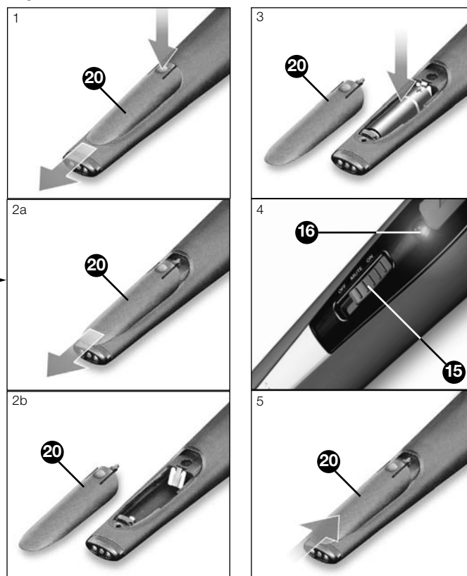
Fig. 8 / HT 40 FLEXX
