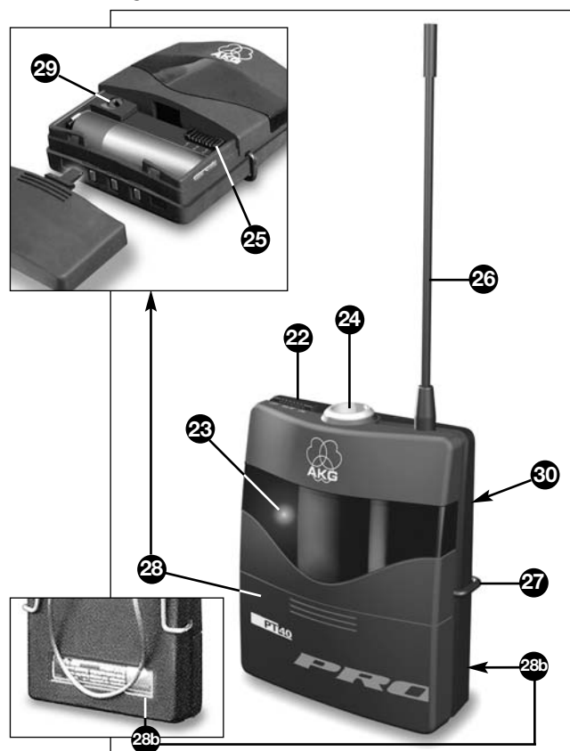
Fig. 4 / PT 40 FLEXX
