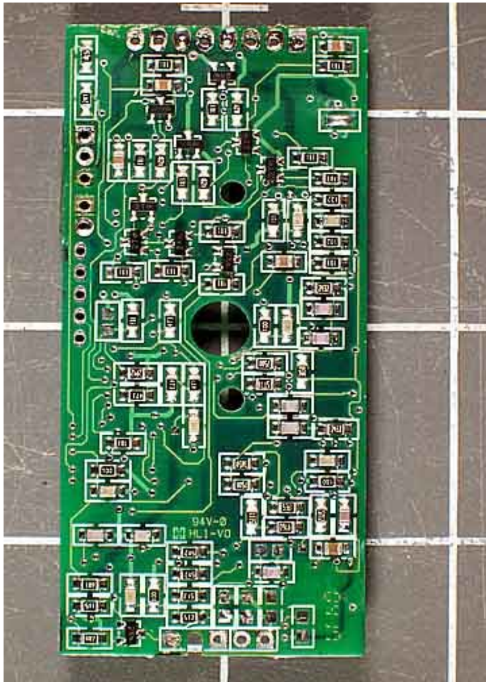
TX PCB Bottom
