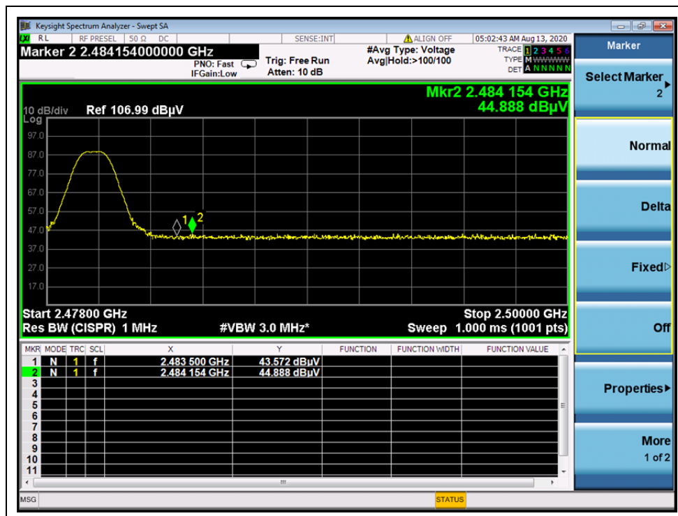
(AVERAGE, Channel 39)
