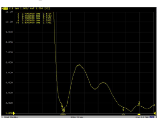
VSWR_BT
