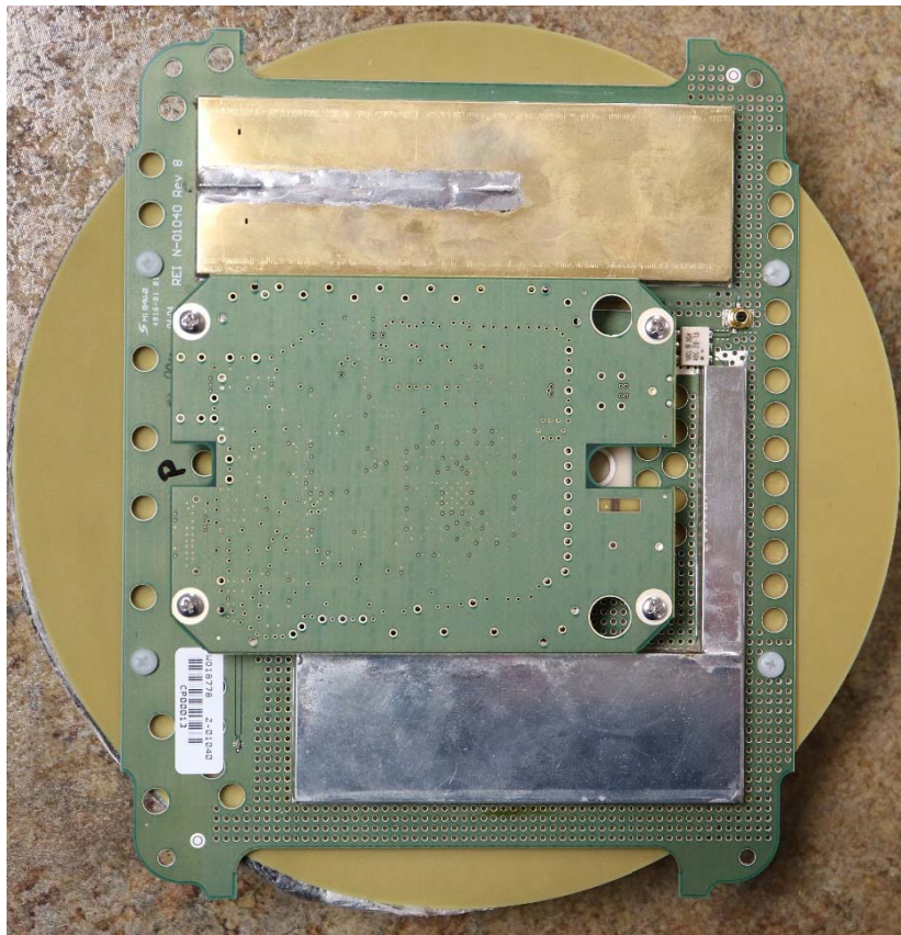
4-00203 ORION 900 ANTENNA / RF BOARD ASSEM– Side A:
