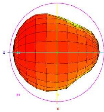
Total_3D_Left View_900MHz
