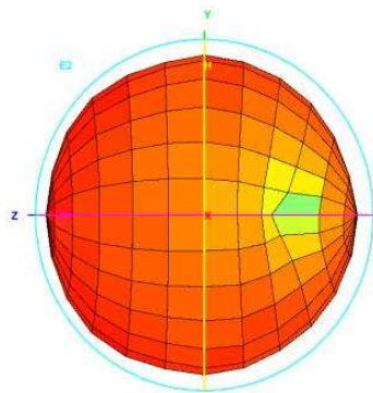
Total_3D_Left View_900MHz
