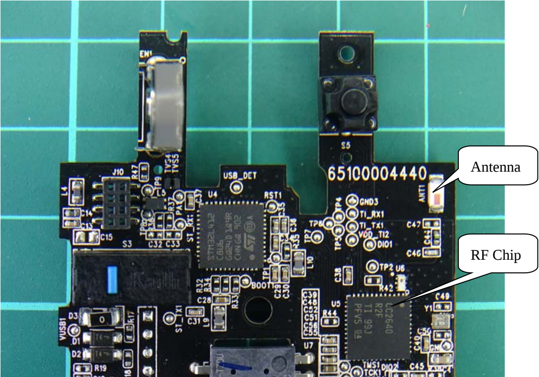
(16) EUT Photo
