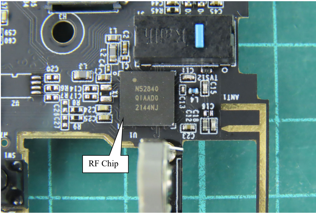
(12) EUT Photo
