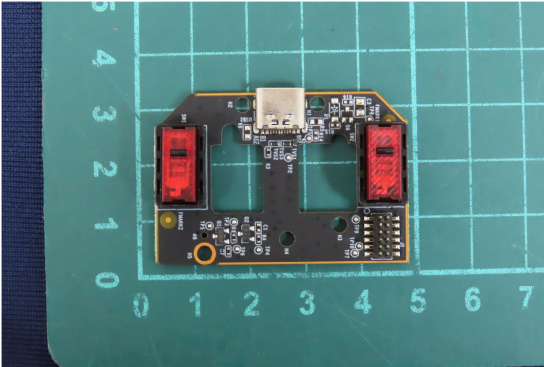
(17) EUT Photo
