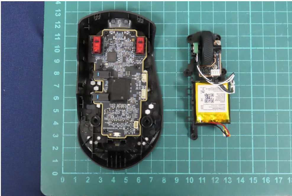
(15) EUT Photo
