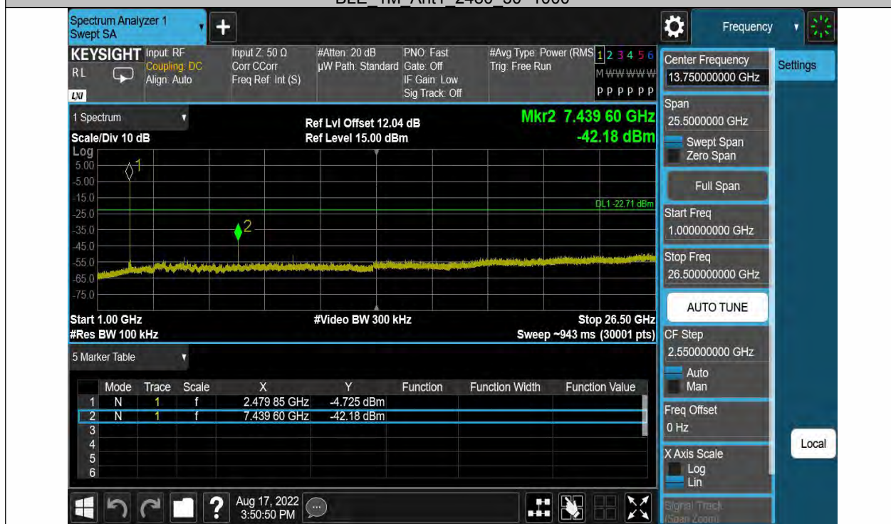
BLE 1M_Ant1_2480_1000~26500
