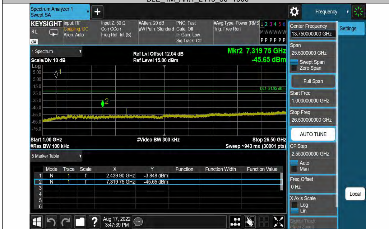
BLE 1M Ant1 2440 1000~26500
