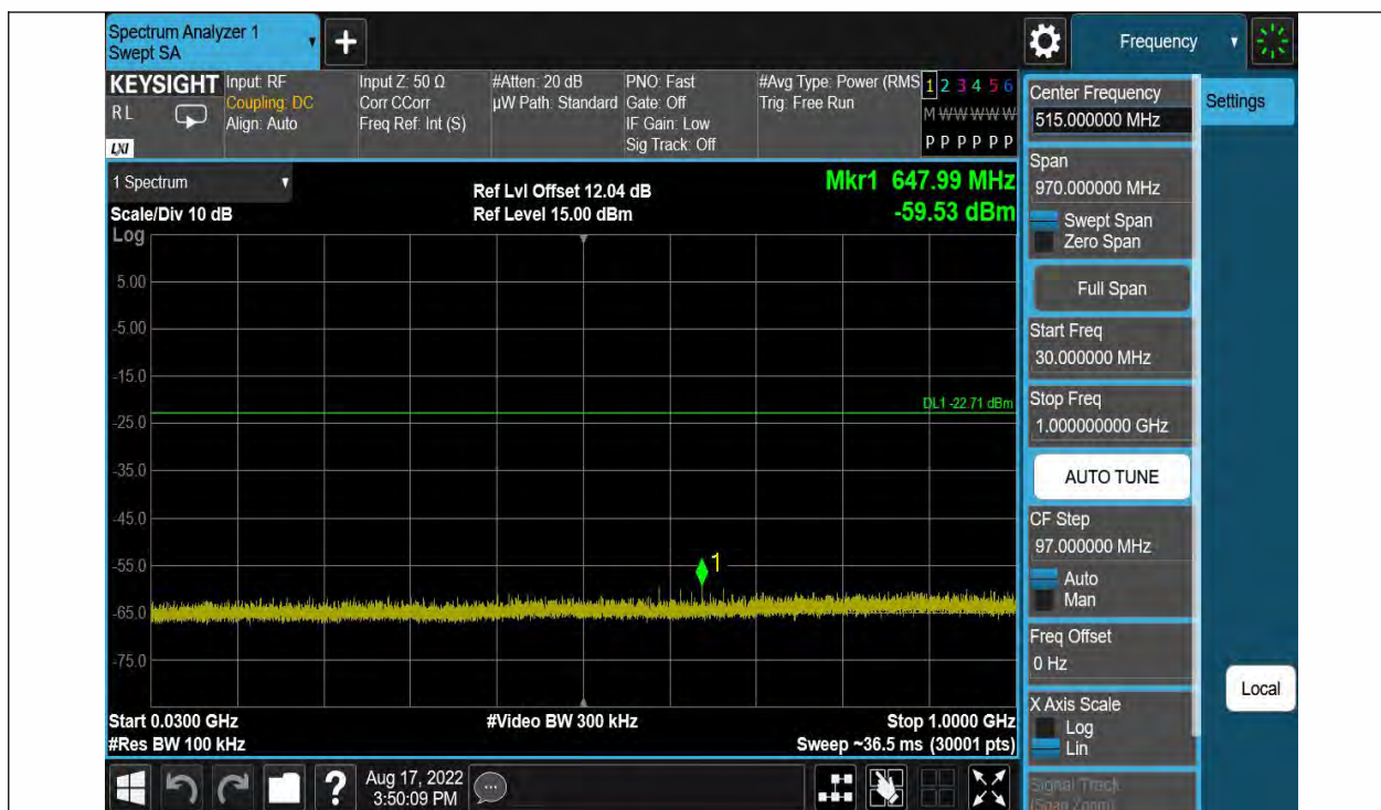
BLE 1M Ant1 2480 30~1000
