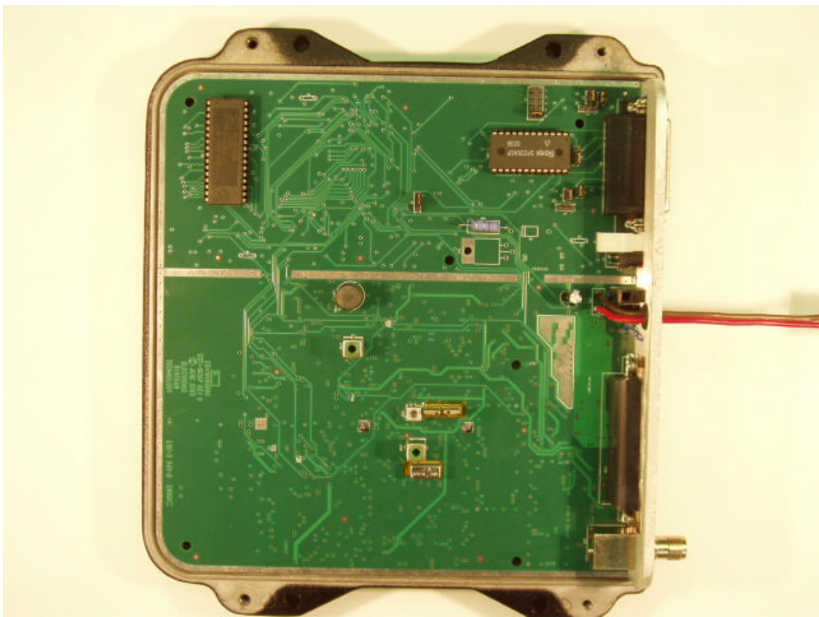
PCB Bottom
