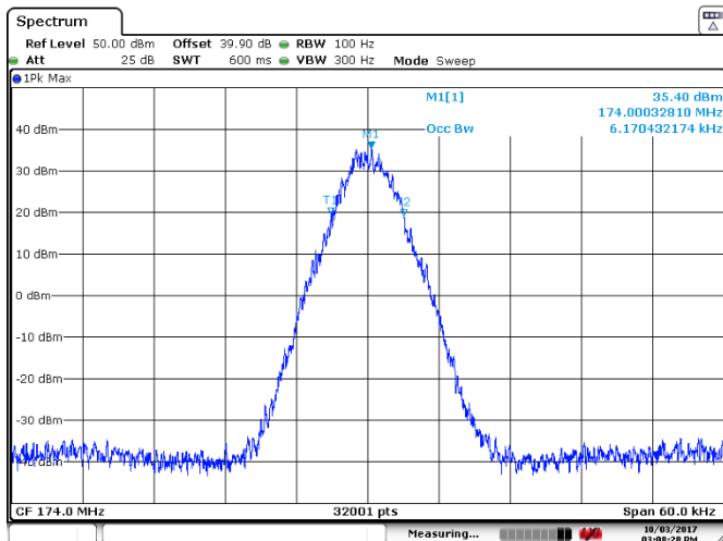
OBW ch174 MHz 12.5KHz dev 2000
